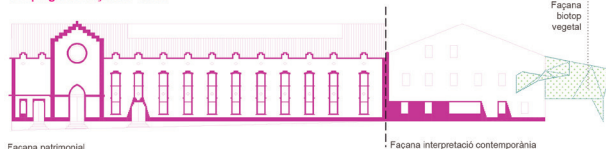
Desplegat de façanes E: 1/500
