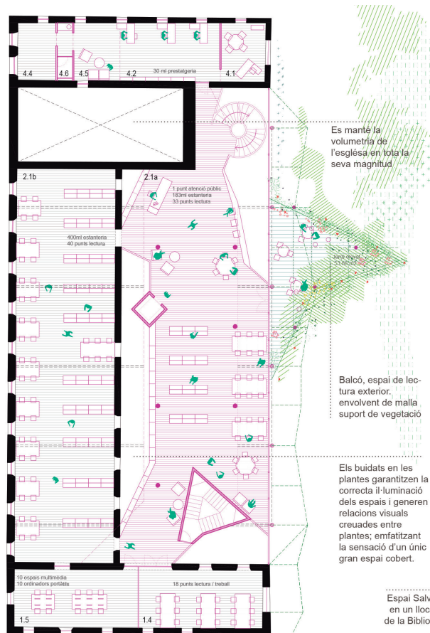
Planta Primera +3.45 E: 1/300
