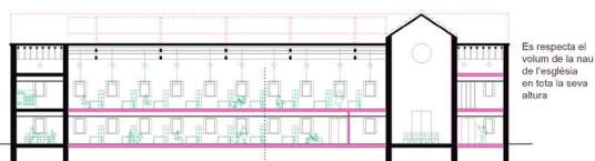
S1. Secció per edifici existent E: 1/400
