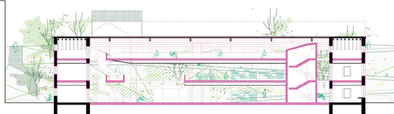
S2. Secció per ampliació E: 1/400
